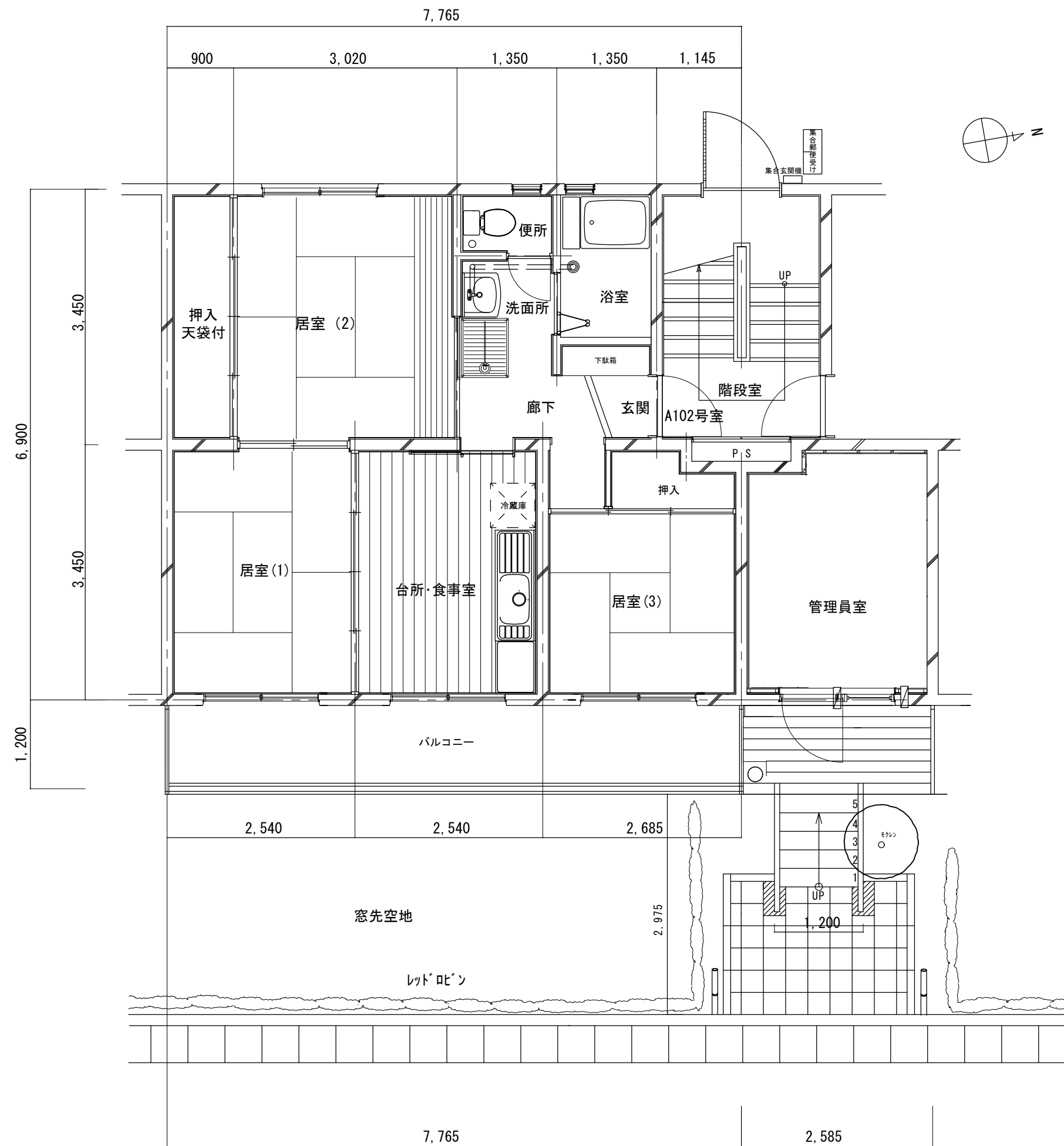
市ヶ谷加賀町アパートA棟102号室平面図
